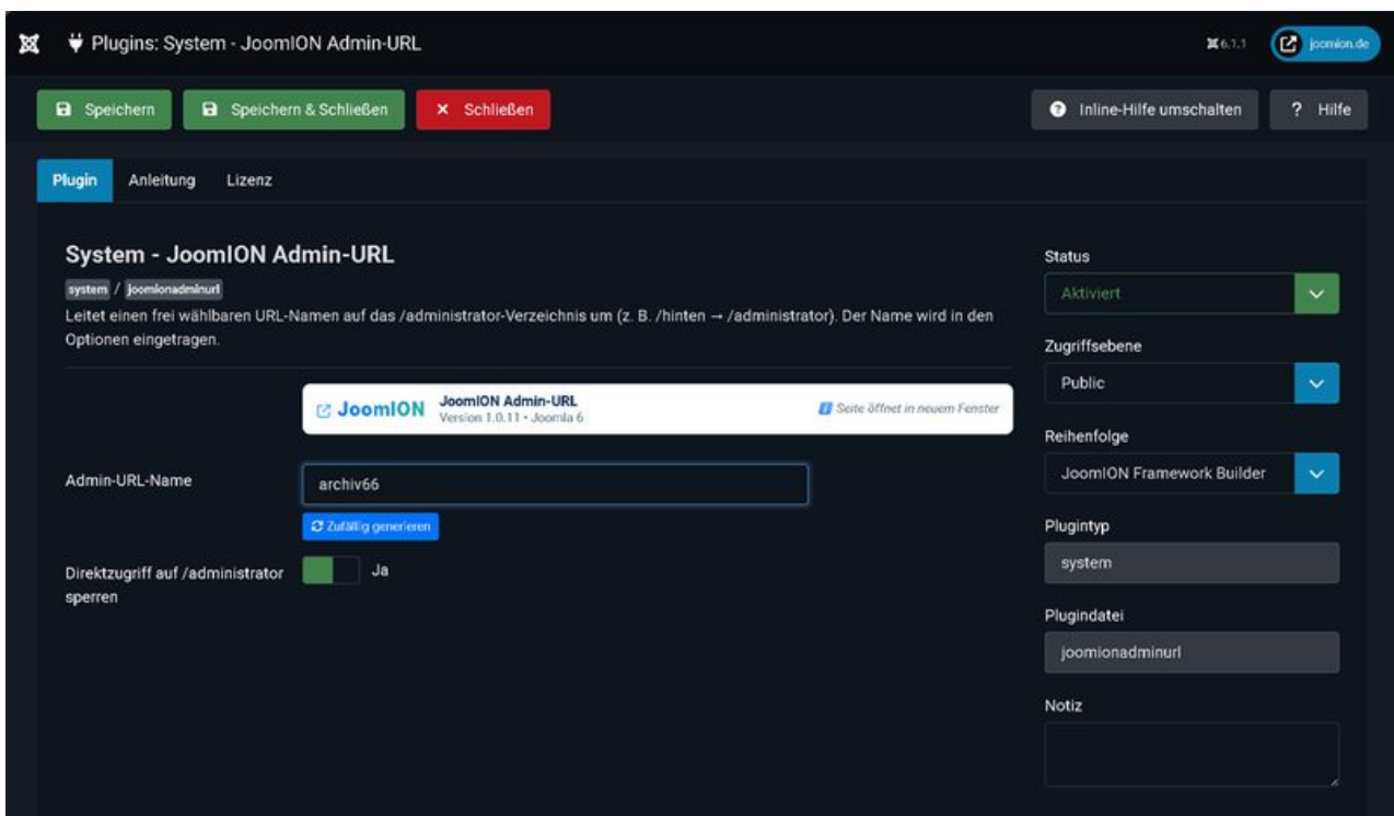
Die Plugin-Einstellungen mit dem Feld „Admin-URL-Name“
